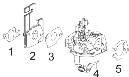
E07 CARBURETOR
