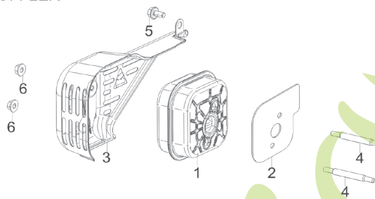
E09 MUFFLER
