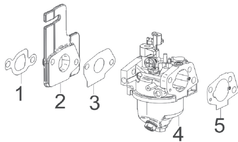
E07 CARBURETOR
